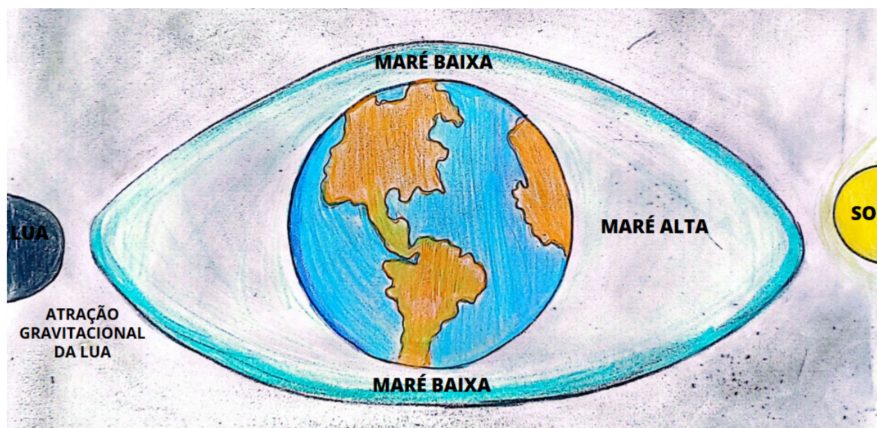
Figura 11- Forma como a Lua e o Sol influenciam nas marés. Fonte: Adaptado de https://gaiaufvjm.blogspot.com/2013/05/como-as-fases-da-lua-influenciam-as.html
