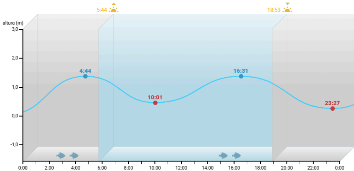
Figura 10. Projeção da tábua das marés com destaque de maré alta (em azul) e maré baixa (em vermelho).
