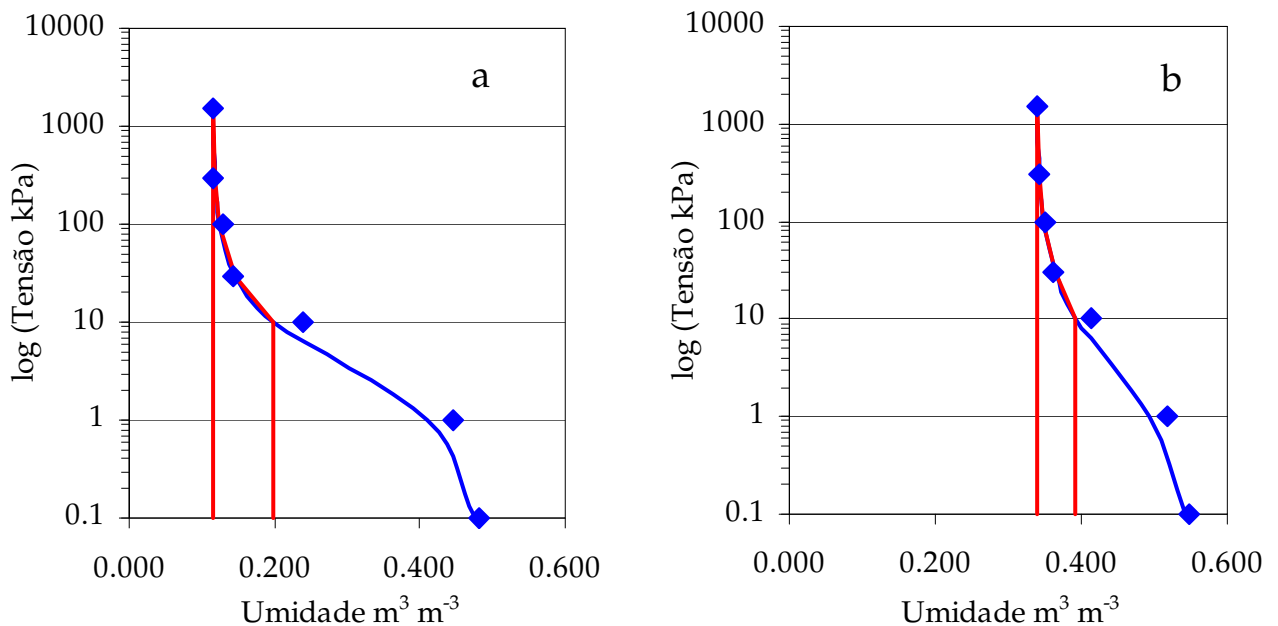
FIGURA 7 – Curva característica da retenção de água no solo, apresentando o volume da água retida ( \text{m}^3 \text{m}^{-3} ) em potenciais de água de 0,1 a 1500 kPa, nos solos (a) LV da topossequência A-B e (b) LVA da topossequência C-D.
