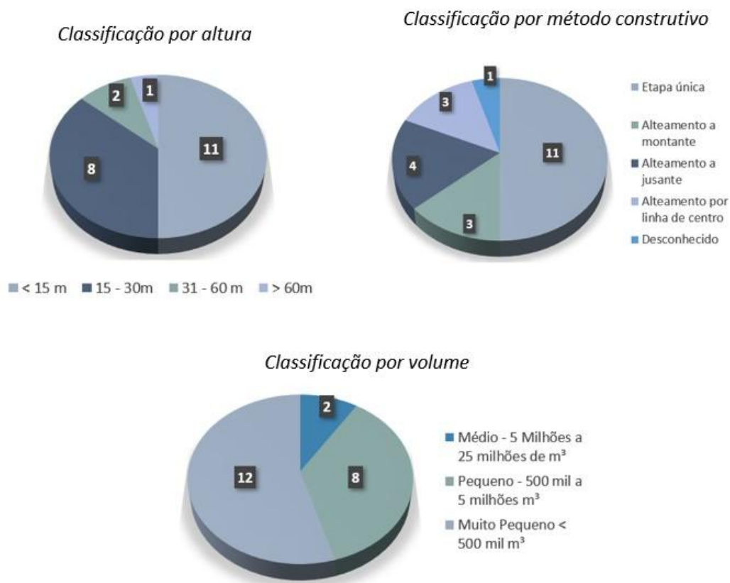
Figura 19: Classificação das barragens de rejeitos de mineração por altura, volume e método construtivo
