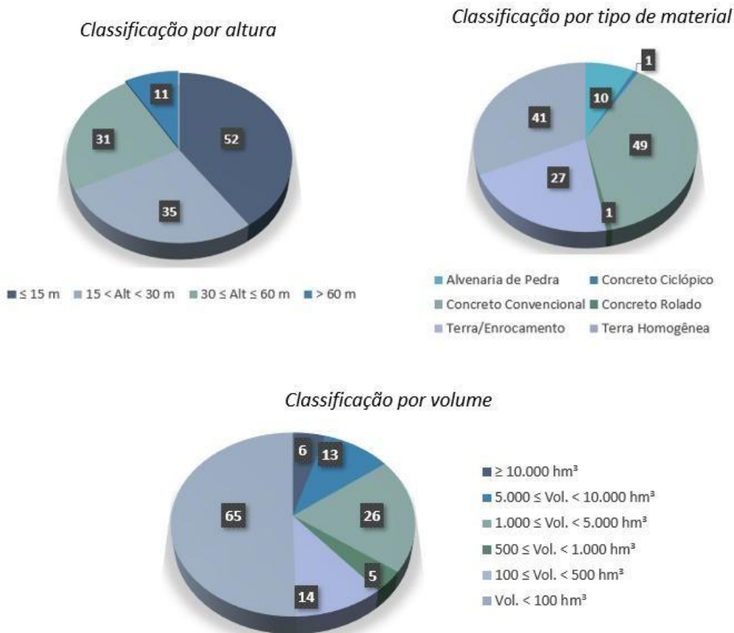
Figura 15: Classificação das barragens de geração de energia elétrica por altura, volume e tipo de material
