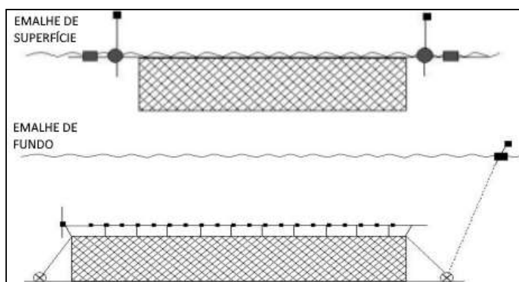
Redes de Emalhe - Fonte: Adaptado de CEPSUL/IBAMA
