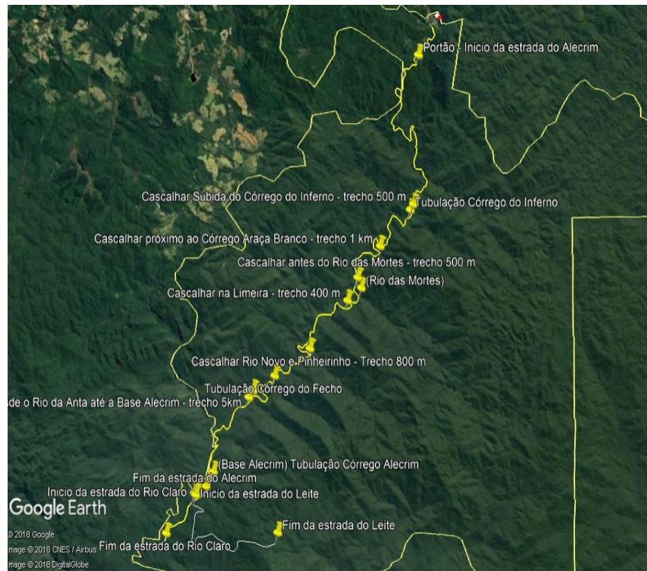
FIGURA 1 – Imagem aérea da estrada Alecrim/Leite. Pontos marcados necessitam da retroescavadeira para colocação da tubulação.
