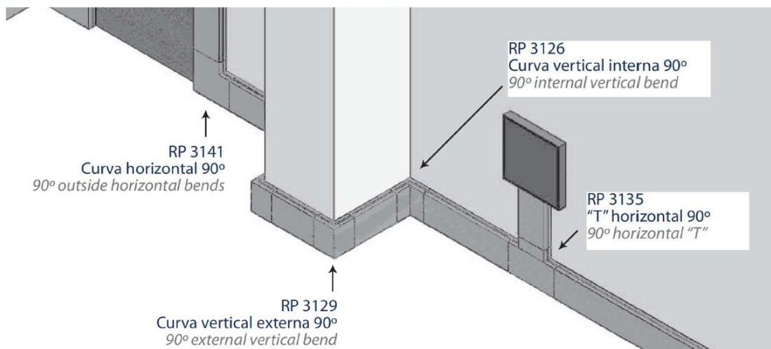
Figura 6 - Exemplo do rodapé e acessórios necessários aos encaminhamentos
