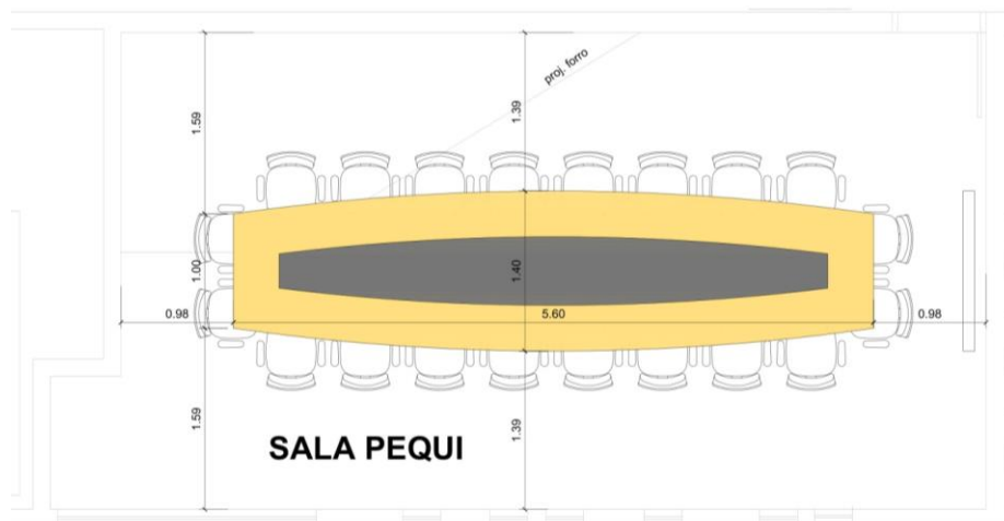
Figura 3 - Layout pretendido para nova sala de reuniões
