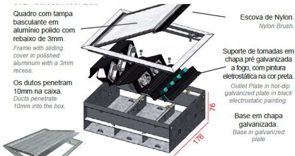
Figura 5 - exemplo da caixa de tomada com tampa basculante
