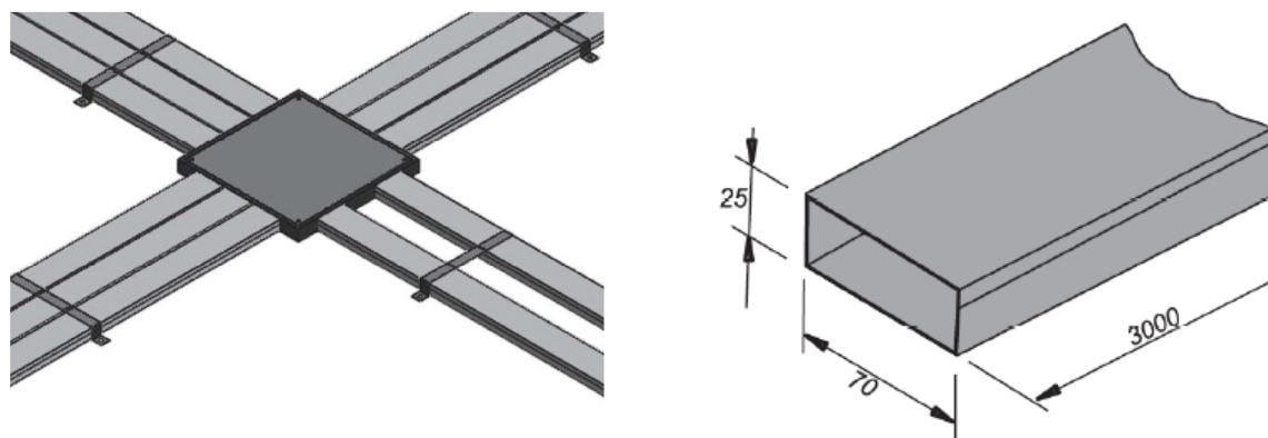
Figura 4 - exemplo do perfil de duto de piso necessário
