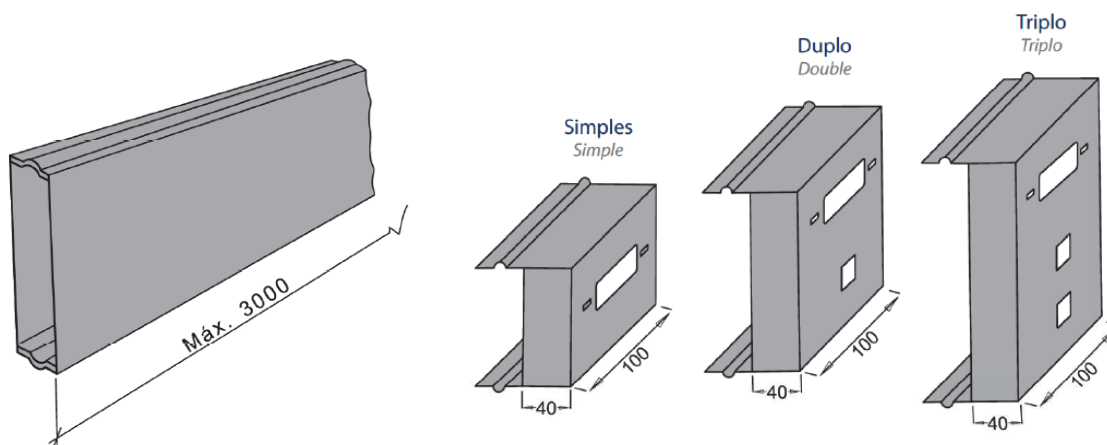
Figura 7 - Detalhe do rodapé e caixas de tomada
