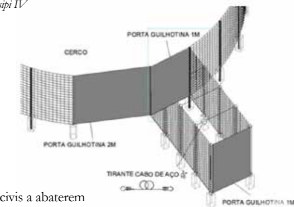
Vista geral do curral de manejo
