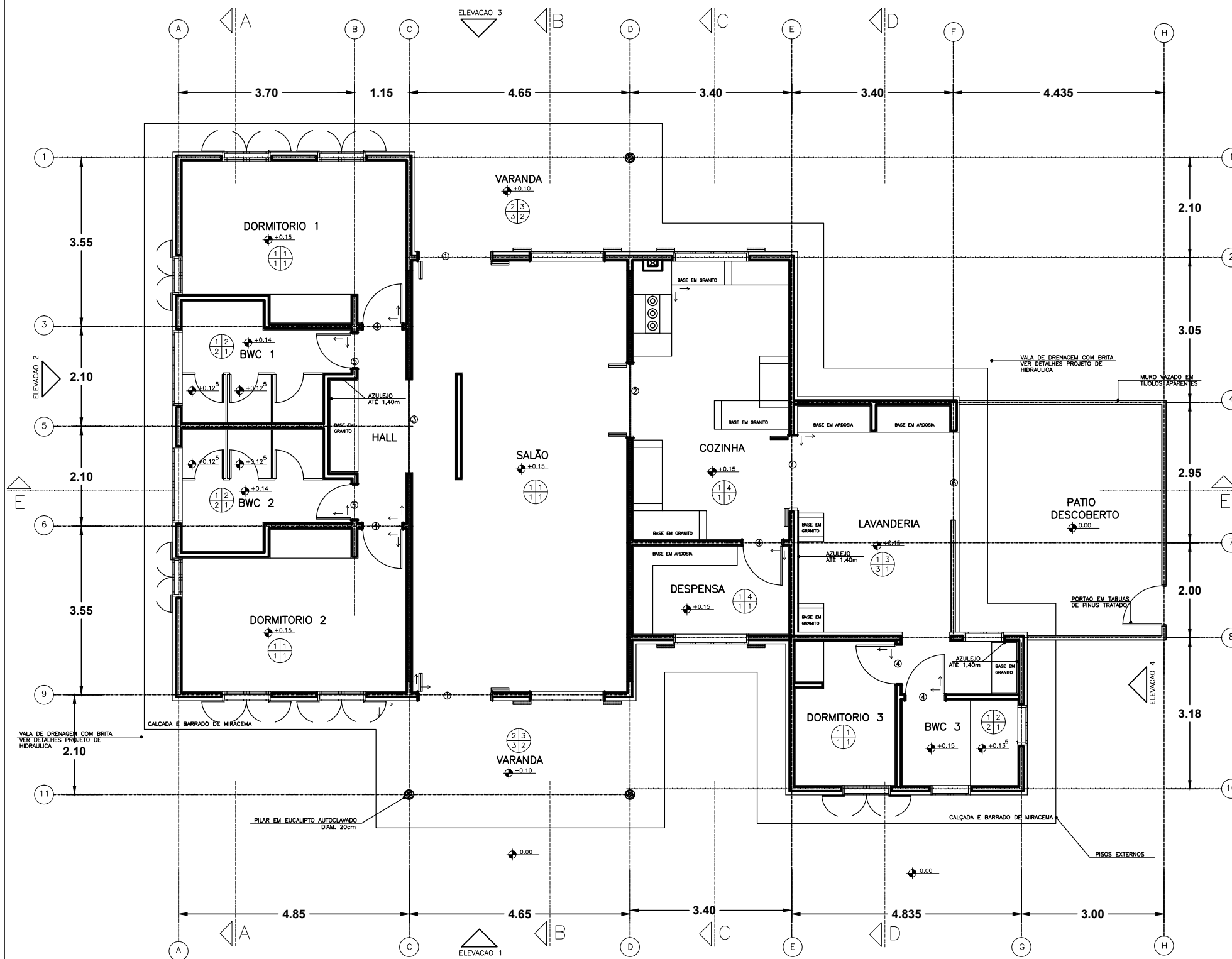
PLANTA DE PISO
