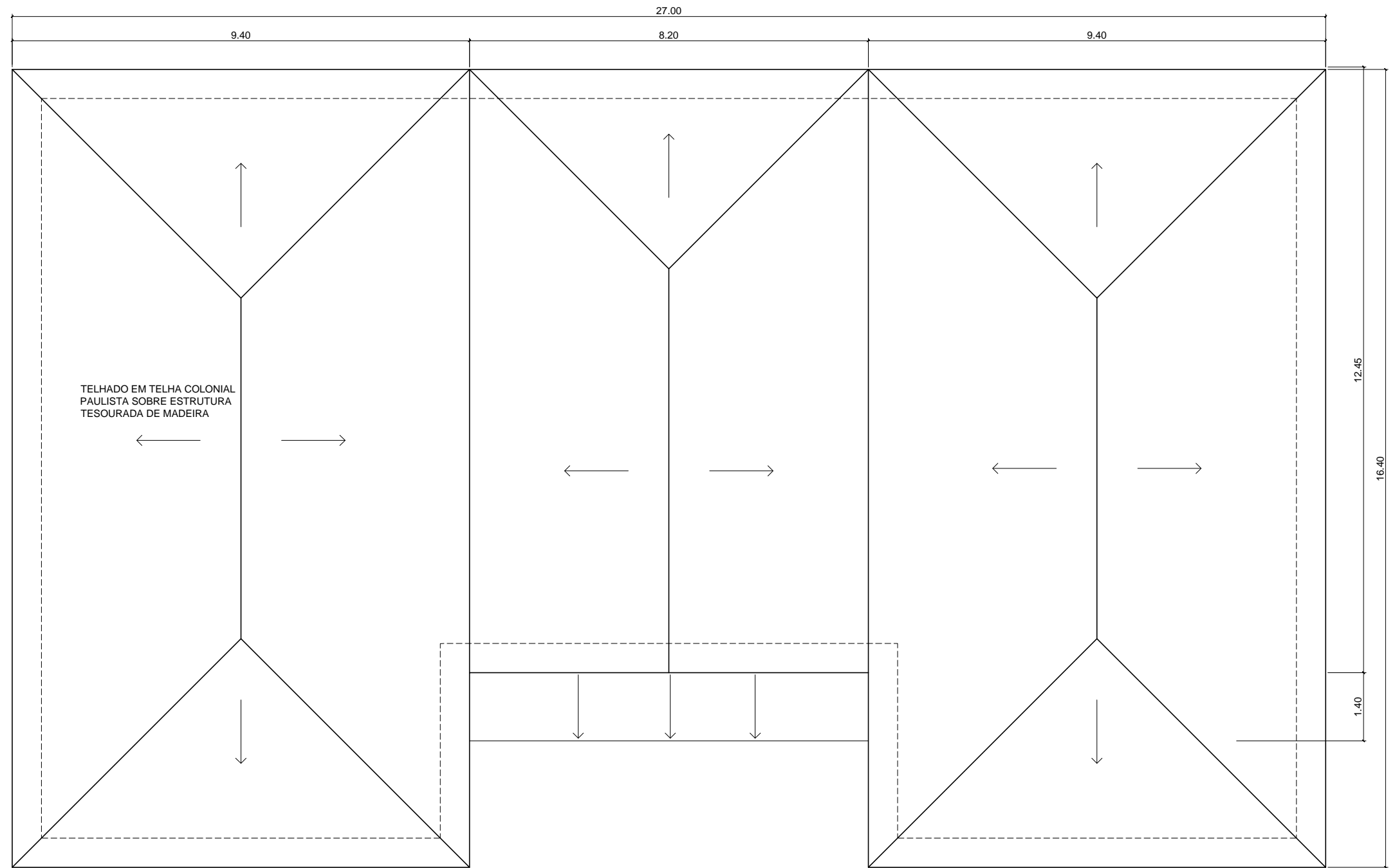
PLANTA DE COBERTURA
