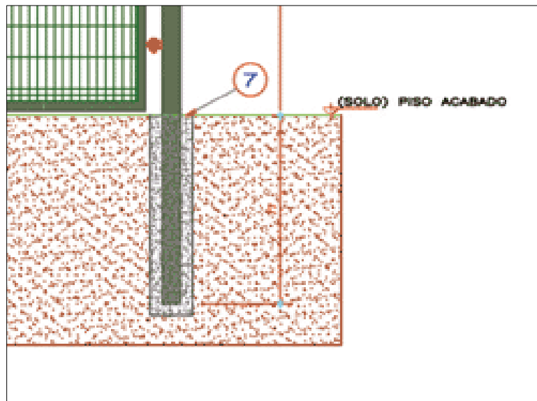
Figura 6 - fixação dos pilaretes com concreto
