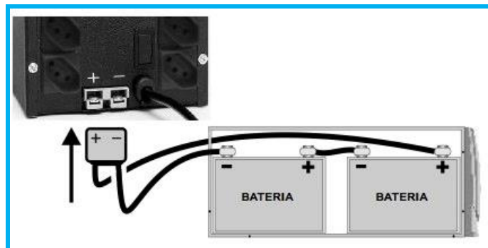
Figura 3 - UPS com Bateria externa.
