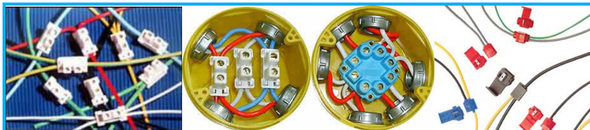
Figura 9 – Conectores e emendas para fios e cabos elétricos.
