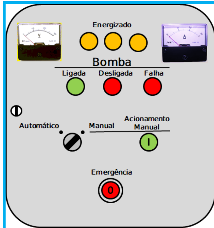
Figura 11 – Frente da caixa de acionamento da bomba.
