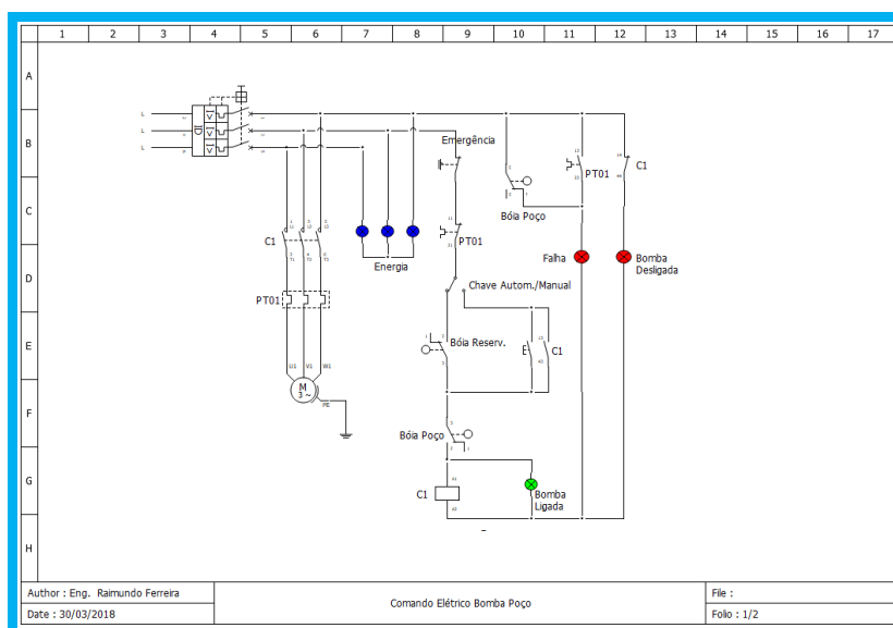
Figura 10 – Esquema de comando elétrico da bomba do poço.
