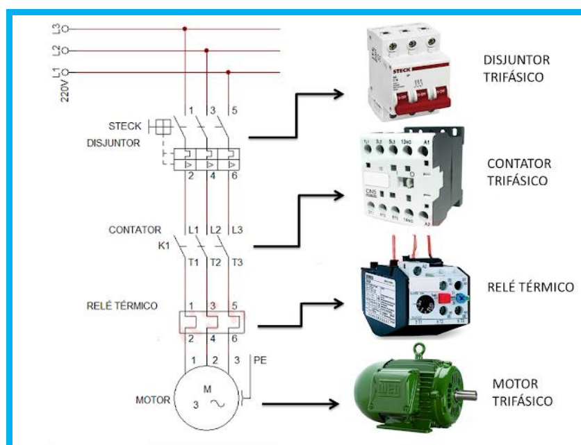
Figura 12 – Exemplo de acionamento de motor.
