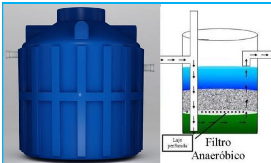
Figura 5 – Filtro Anaeróbico.
