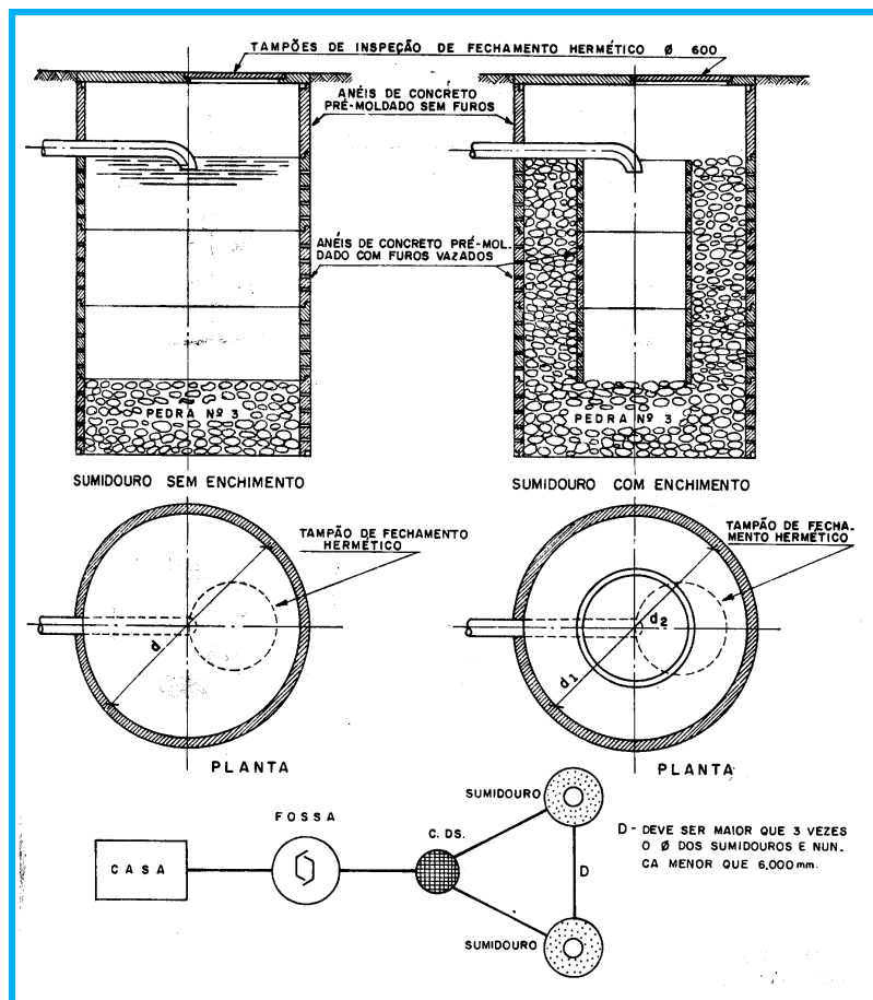
Figura 10 – Detalhe de construção de um sumidouro conforme norma NBR 13969.
