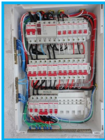
Figura 5 - Quadro de distribuição com pente de borne.
