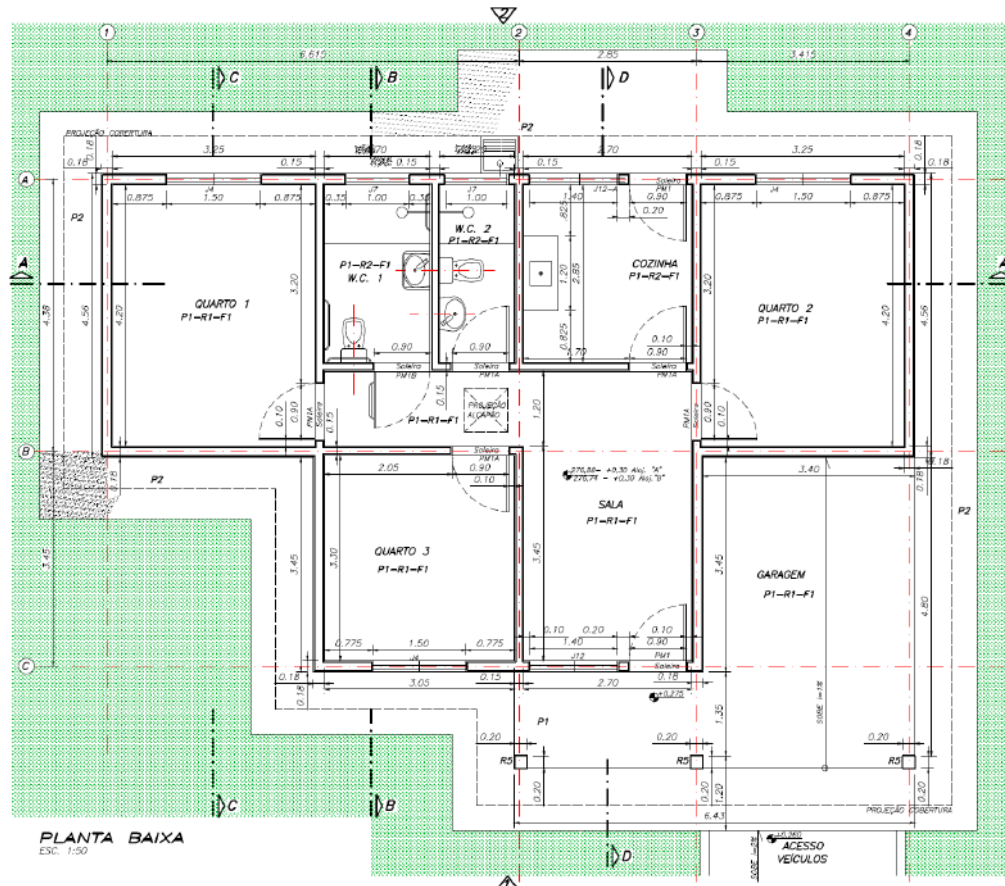
Figura 3 – Planta do Alojamento
