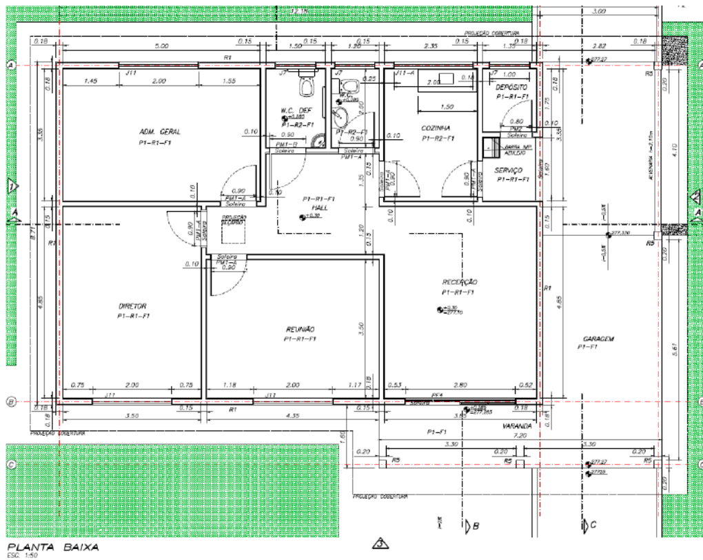
FIGURA 1 – Planta da Administração
