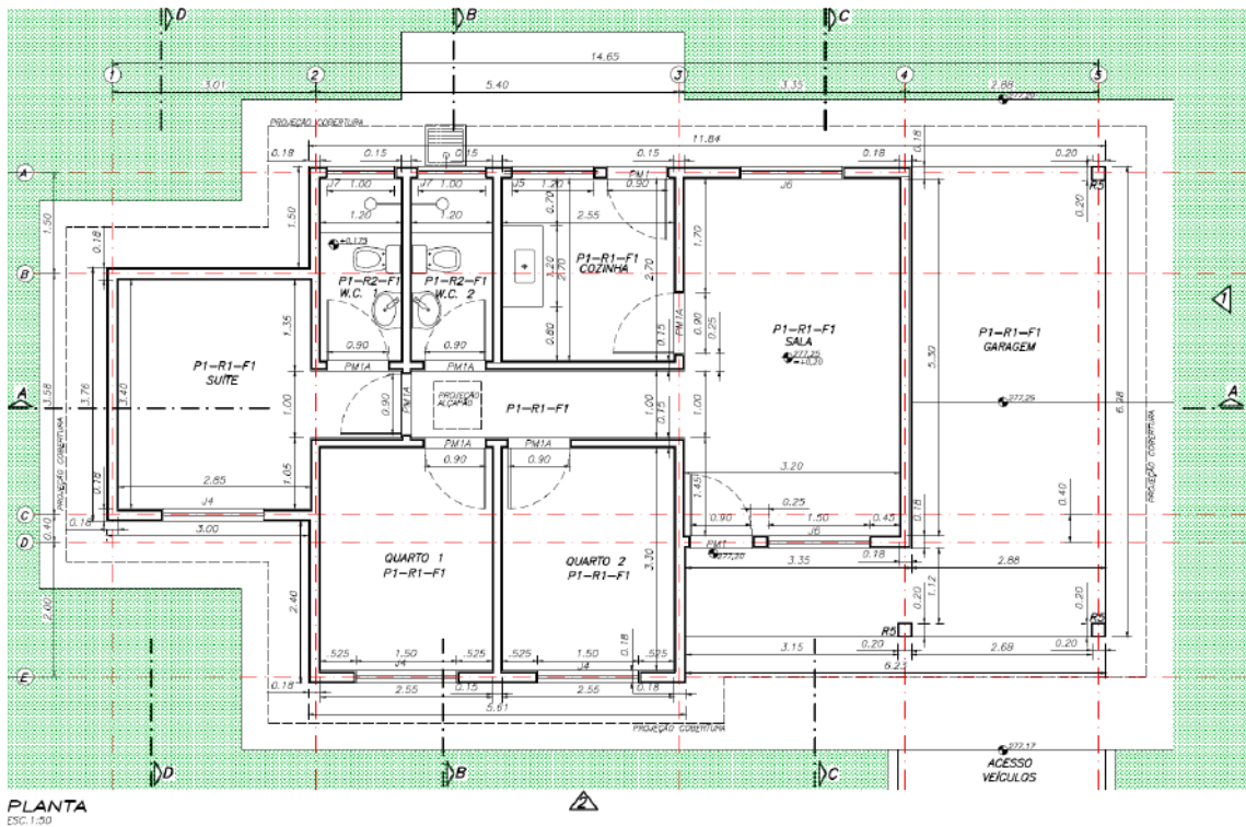
Figura 2 – Planta da Zeladoria
