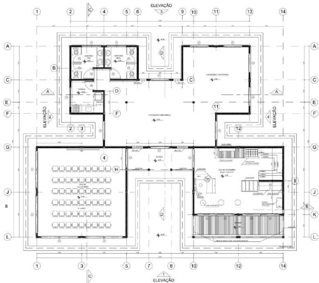
Figura 4 – Planta do Centro de Visitantes
