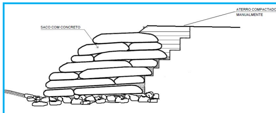
Figura 4 - Forma de assentamento das bolsas de concreto.
