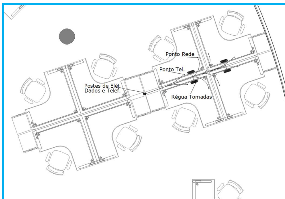
Figura 9 - Exemplo de instalação de infraestrutura nas mesas.
