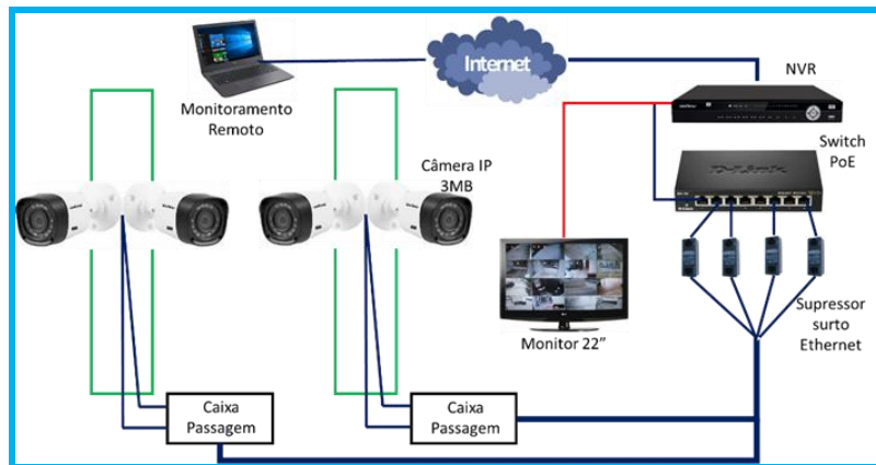
Figura 8 – Esquema de ligação dos equipamentos.
