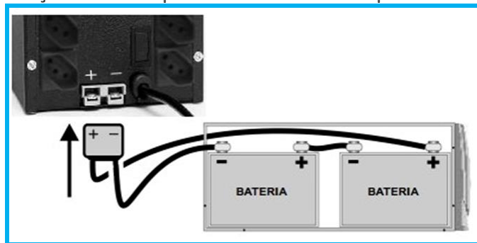
Figura 7 – Exemplo de ups com bateria externa.
