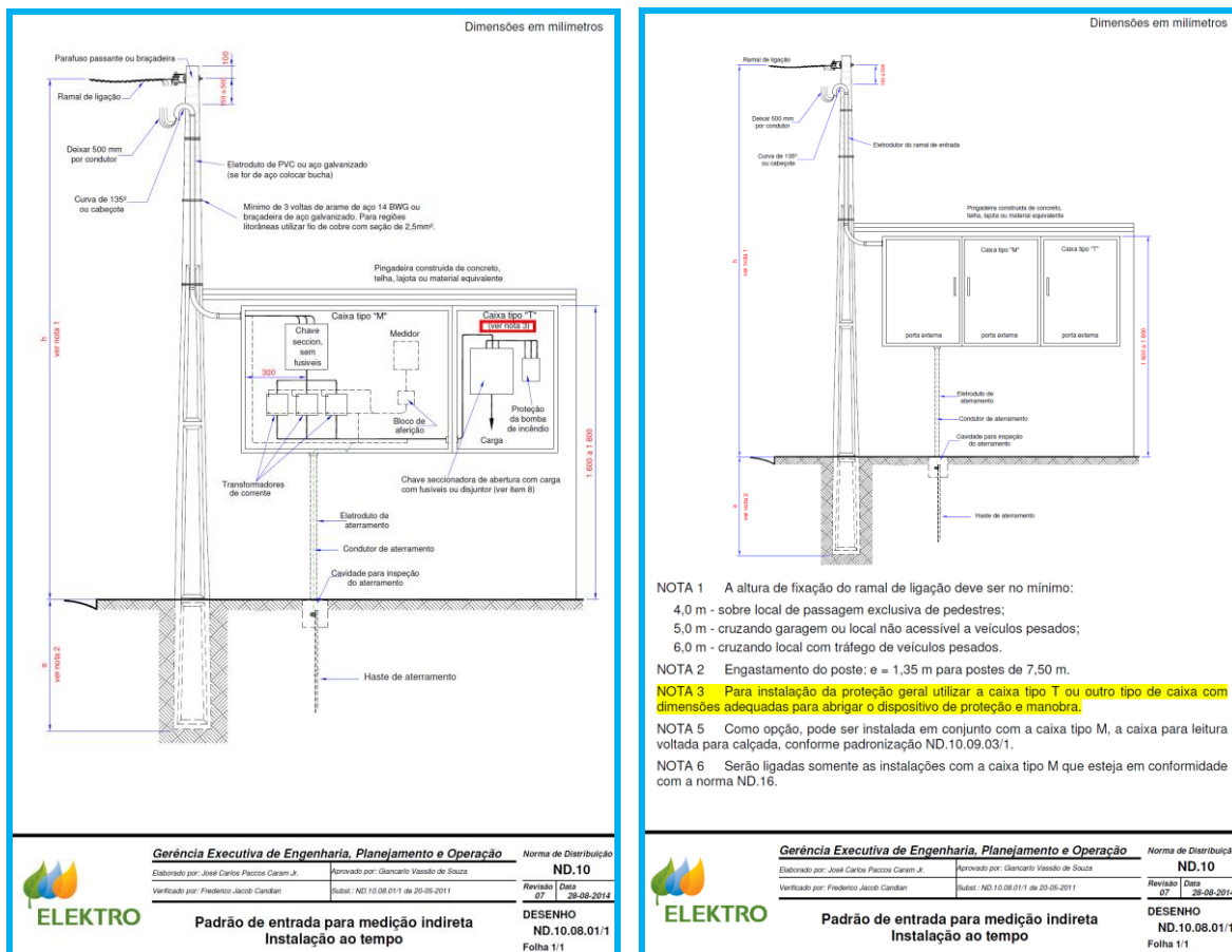
Figura 3 - Padrão de entrada de energia das páginas do manual ND.10 - Elektro.
