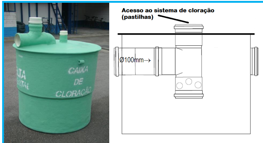
Figura 9 – Exemplo de caixa de cloração em fibra de vidro.
