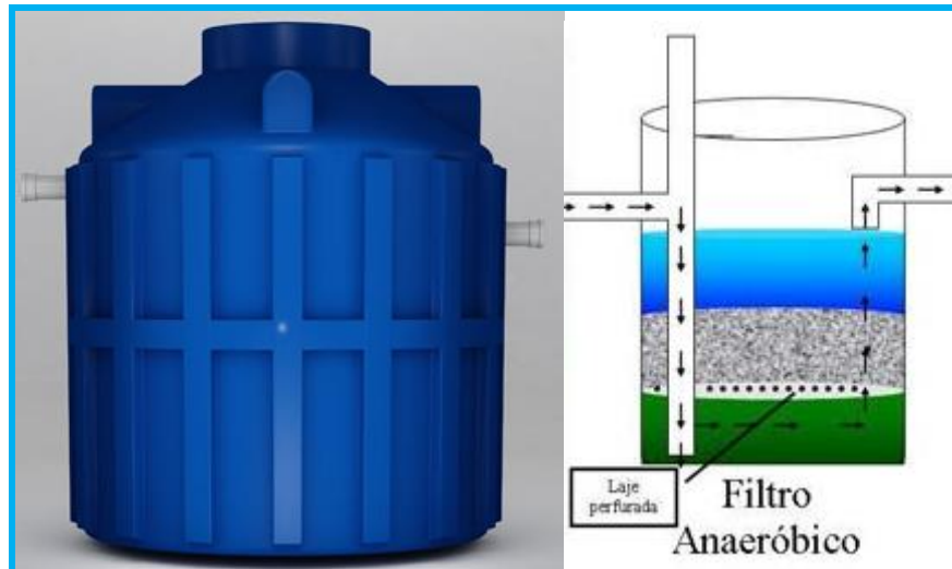
Figura 5 – Filtro Anaeróbio.
