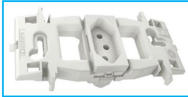
Figura 6 – Tomadas e interruptores em módulos para condutele.
