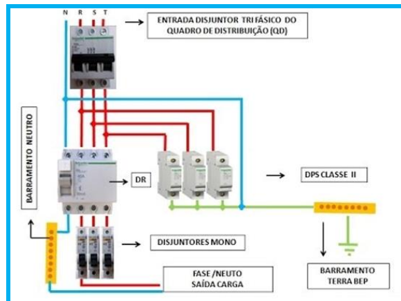
Figura 3 – Dispositivo DR para ligação FFN.
