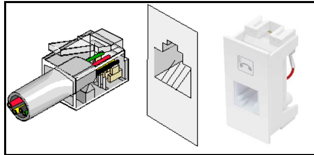
Figura 20 – Conectores e tomada tipo RJ11 para telefonia.
