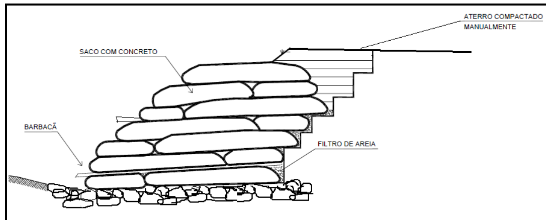
Figura 4 - Forma de assentamento das bolsas de concreto.
