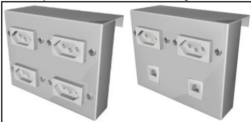
Figura 9 – Suporte para tomadas em metal encaixável em canaleta metálica.
