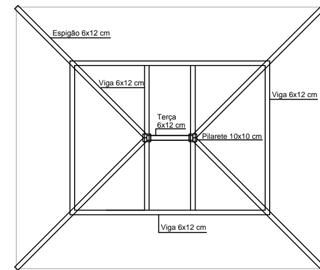
SANITÁRIO PROPOSTA ESTRUTURA DO TELHADO 1:50
