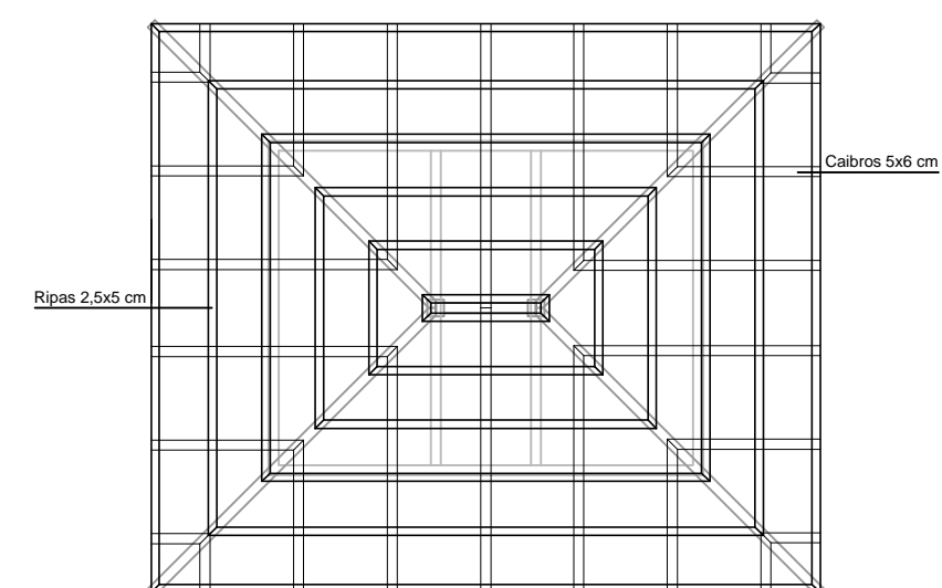
SANITÁRIO PROPOSTA ESTRUTURA DO TELHADO 1:50
