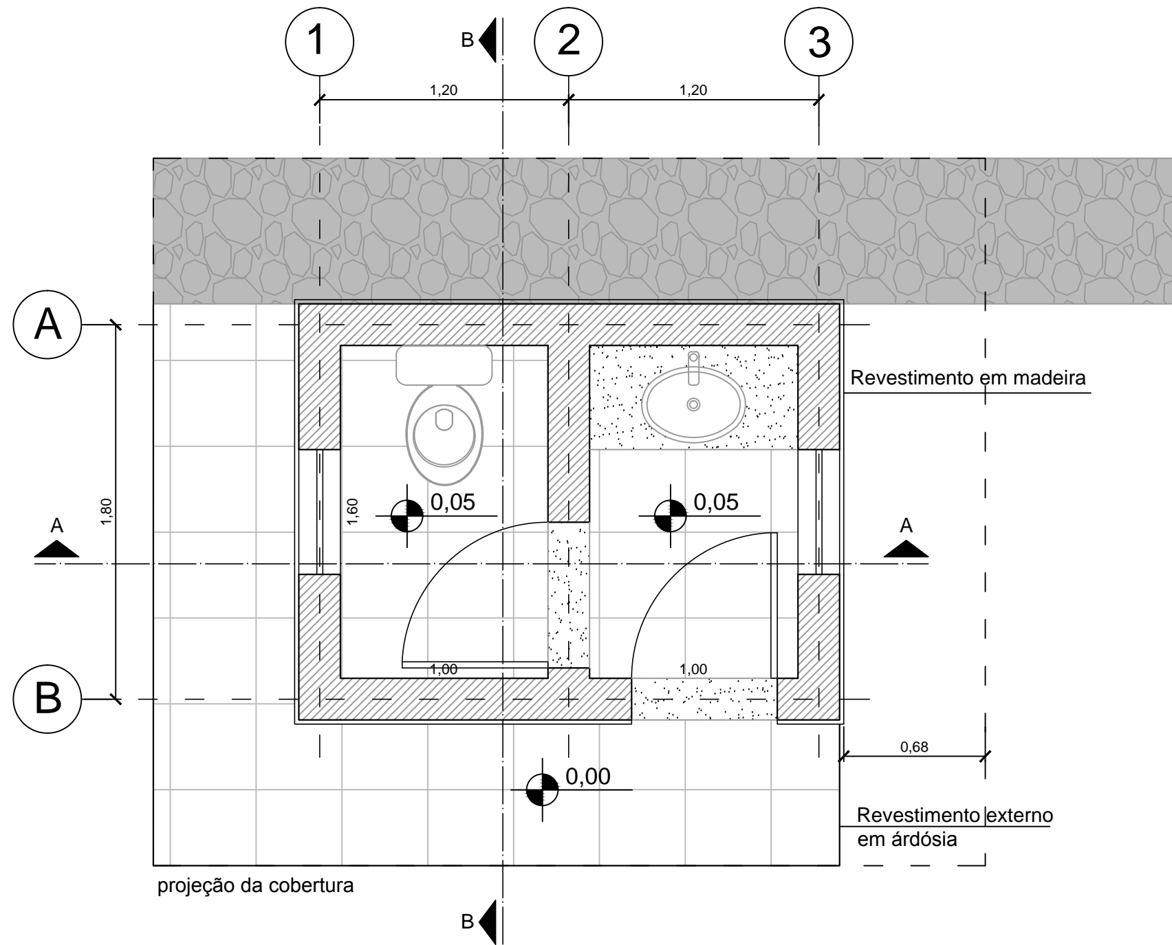
SANITÁRIO PROPOSTA PLANTA
