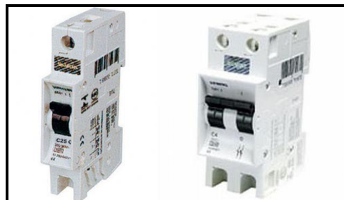
Figura 16 – Disjuntor monopolar e bipolar padrão DIN.
