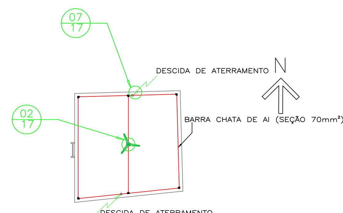
PLANTA COBERTURA CAIXA D'ÁGUA ESCALA 1:100
