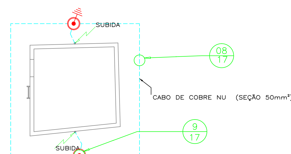
PLANTA BAIXA CAIXA D'ÁGUA ESCALA 1:100
