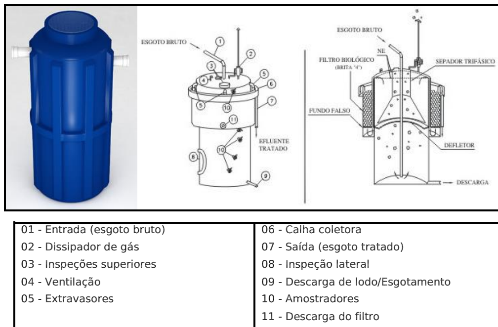
Figura 4 – Reator Anaeróbio.
