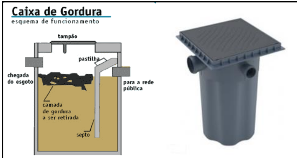
Figura 6 – Exemplo de caixa de gordura.
