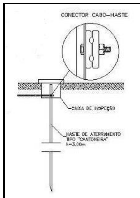
Figura 10 – Sistema de aterramento.
