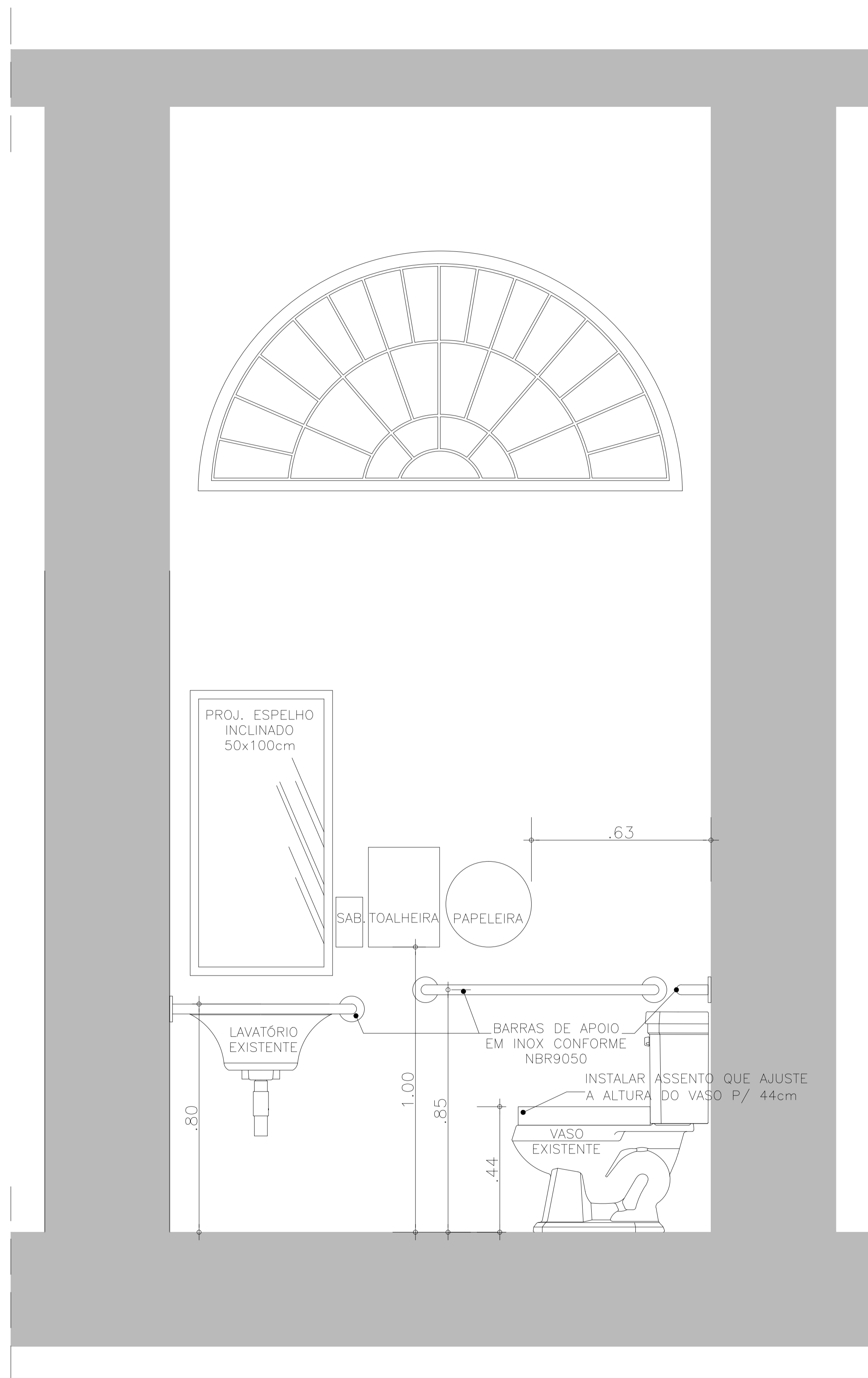
CORTE C – ESQUEMÁTICO ESTRUTURAL – LAVABO ACESSÍVEL – PAVIMENTO TÉRREO ESCALA 1:20
