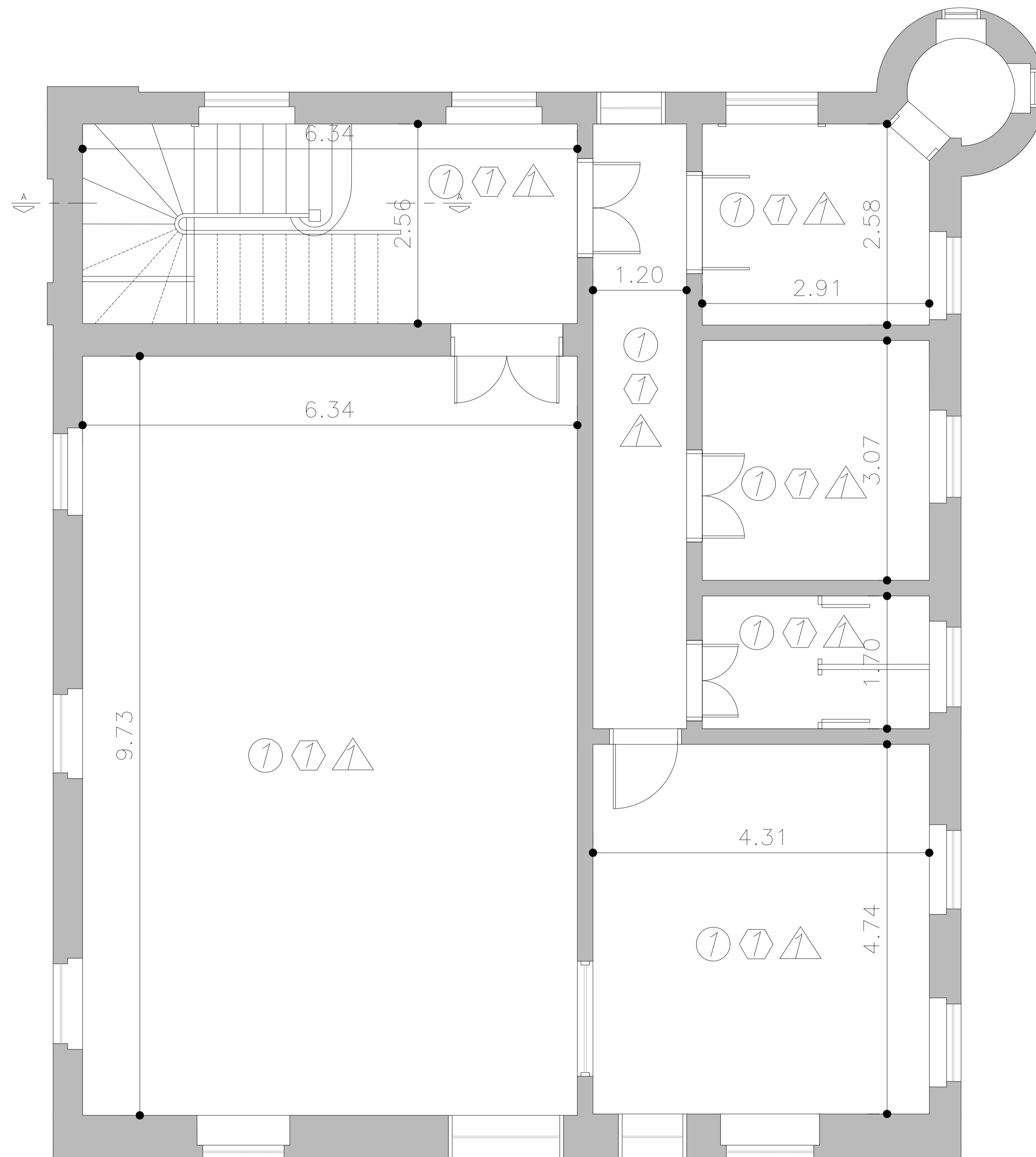
Planta de relação de serviços Pav. Superior Escala 1:75
