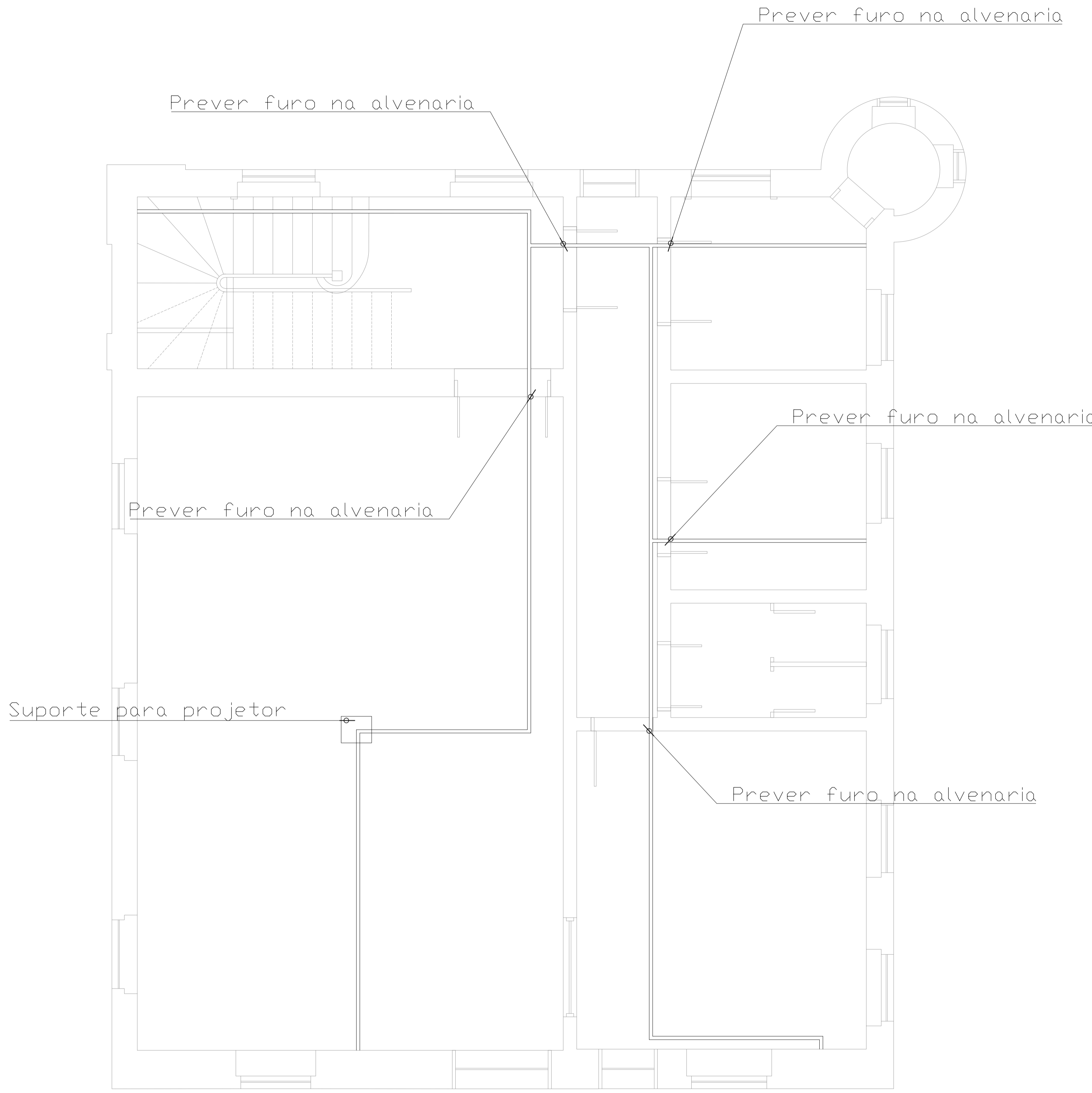
Planta de passagem de eletrocalha para lógica Escala 1:75
