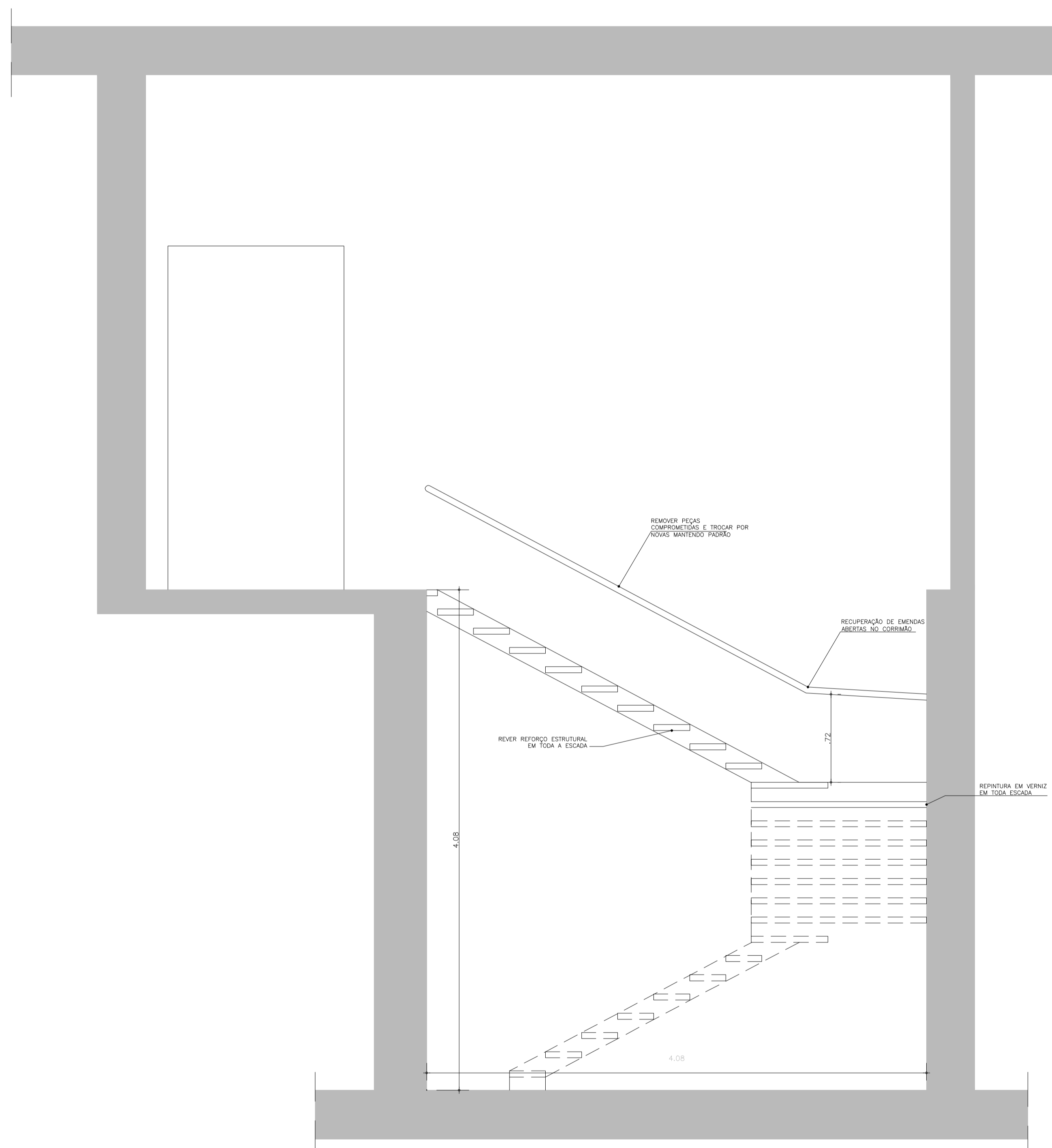
CORTE A ESCADA DE MADEIRA PARA RESTAURO E REFORÇO ESTRUTURAL ESCALA: 1:20
