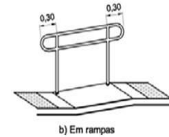
Detalhe dos Corrimãos
