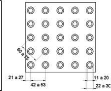
Figura 2 – Piso tátil de Alerta 25x25cm
