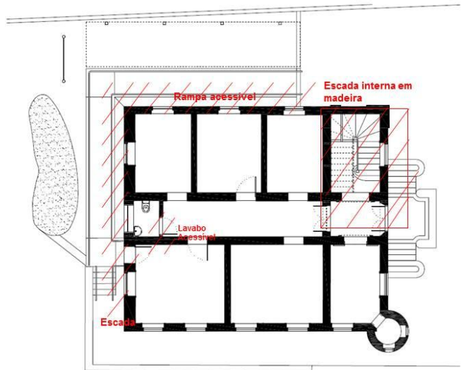
Planta Pavimento Térreo Sem Escala
