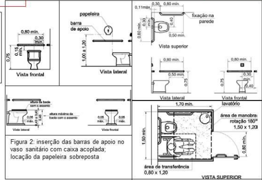
DIMENSIONAMENTO DAS BARRAS DE APOIO
