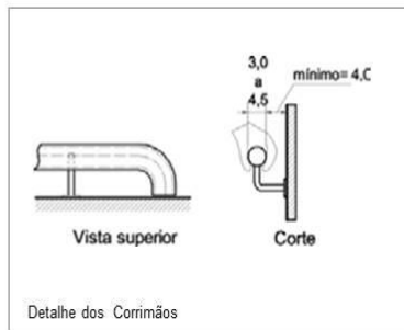
Detalhe dos Corrimãos
