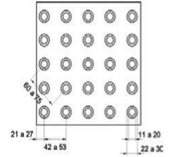
Figura 3 – Piso tátil de Alerta 25x25cm
