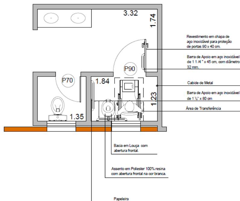
PLANTA DO SANITÁRIO ACESSÍVEL ESC: 1:50
