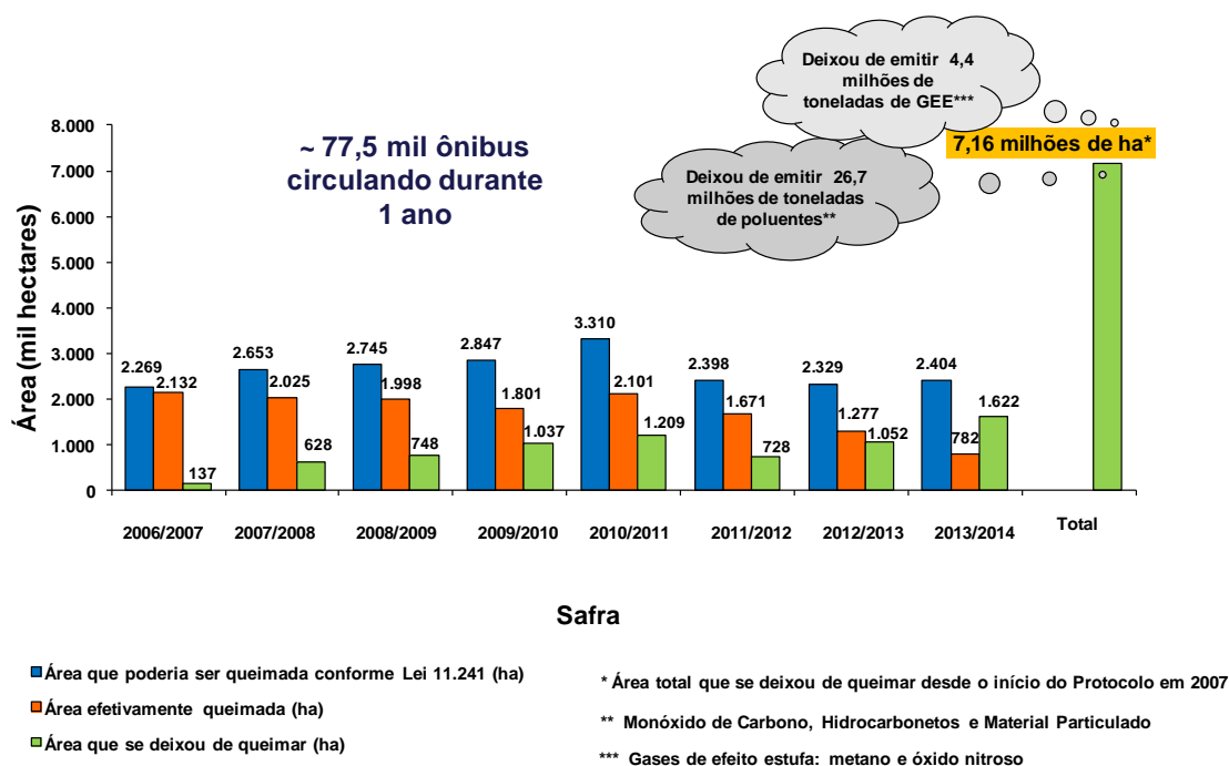
Figura 26 - Ganhos Ambientais com a Redução da Queima, Estado de São Paulo, 2006/07 a 2013/14.
