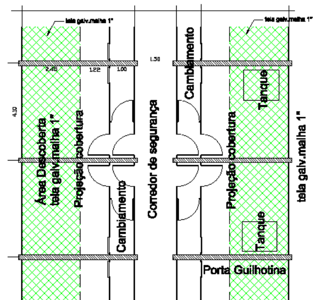
CETAS REGISTRO ESTRUTURA BÁSICA - RECINTOS Sem escala
