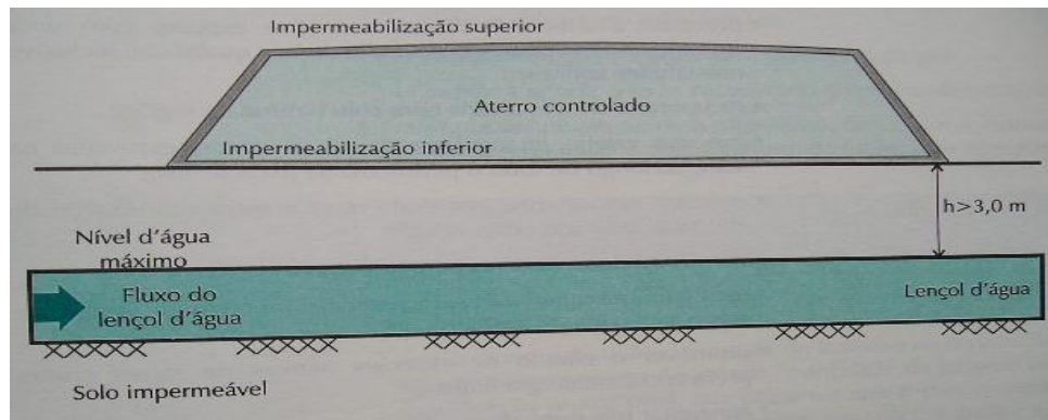
Figura 4. Esquema do aterro controlado.
