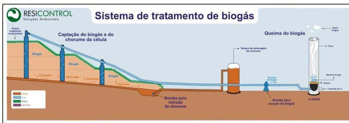
Figura 3.3.1.3.10 - Sistema de Tratamento de Biogás
