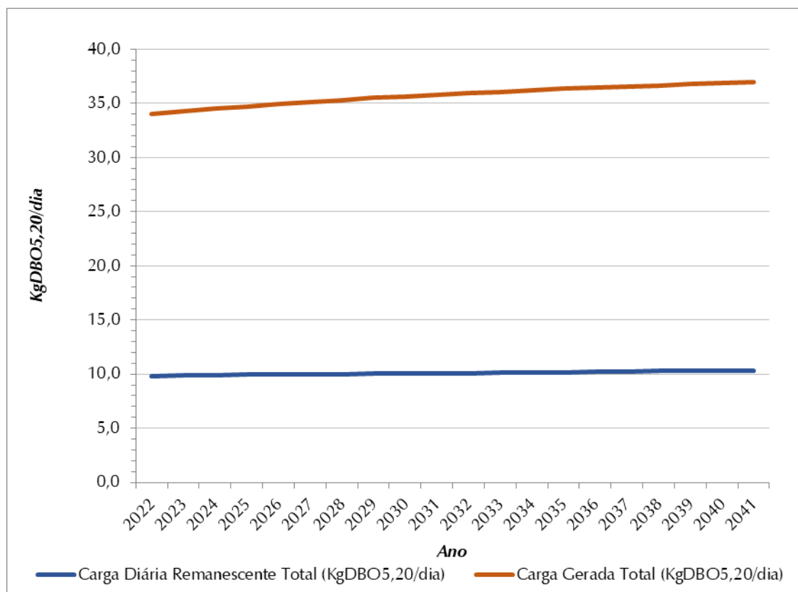
Figura 8.8 - Evolução de Cargas Orgânicas (Kg DBO 5,20 /Dia) – SES Juritis
