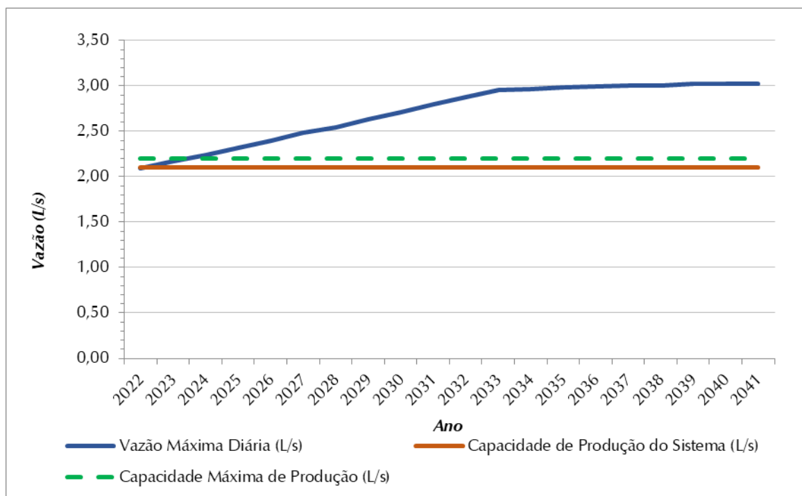
Figura 8.3 – Demandas Máximas Diárias (L/s) X Vazão Captada (L/s) – SAA Juritis
