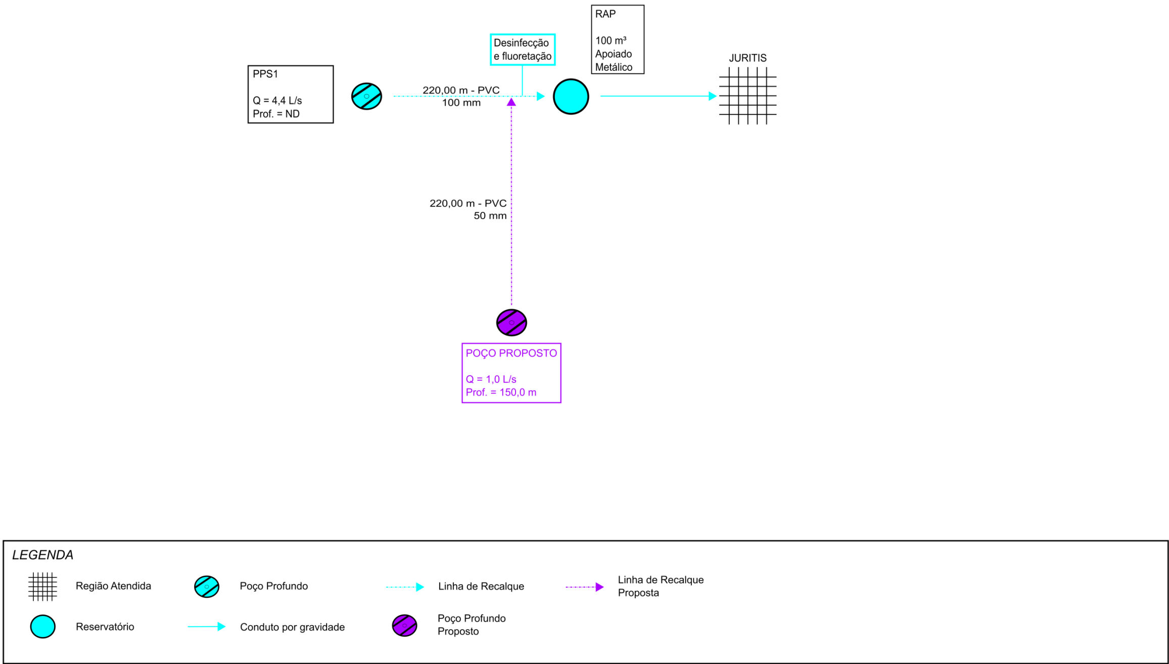
Figura 10.2 – Croqui das intervenções propostas no sistema de abastecimento de água Juritis
