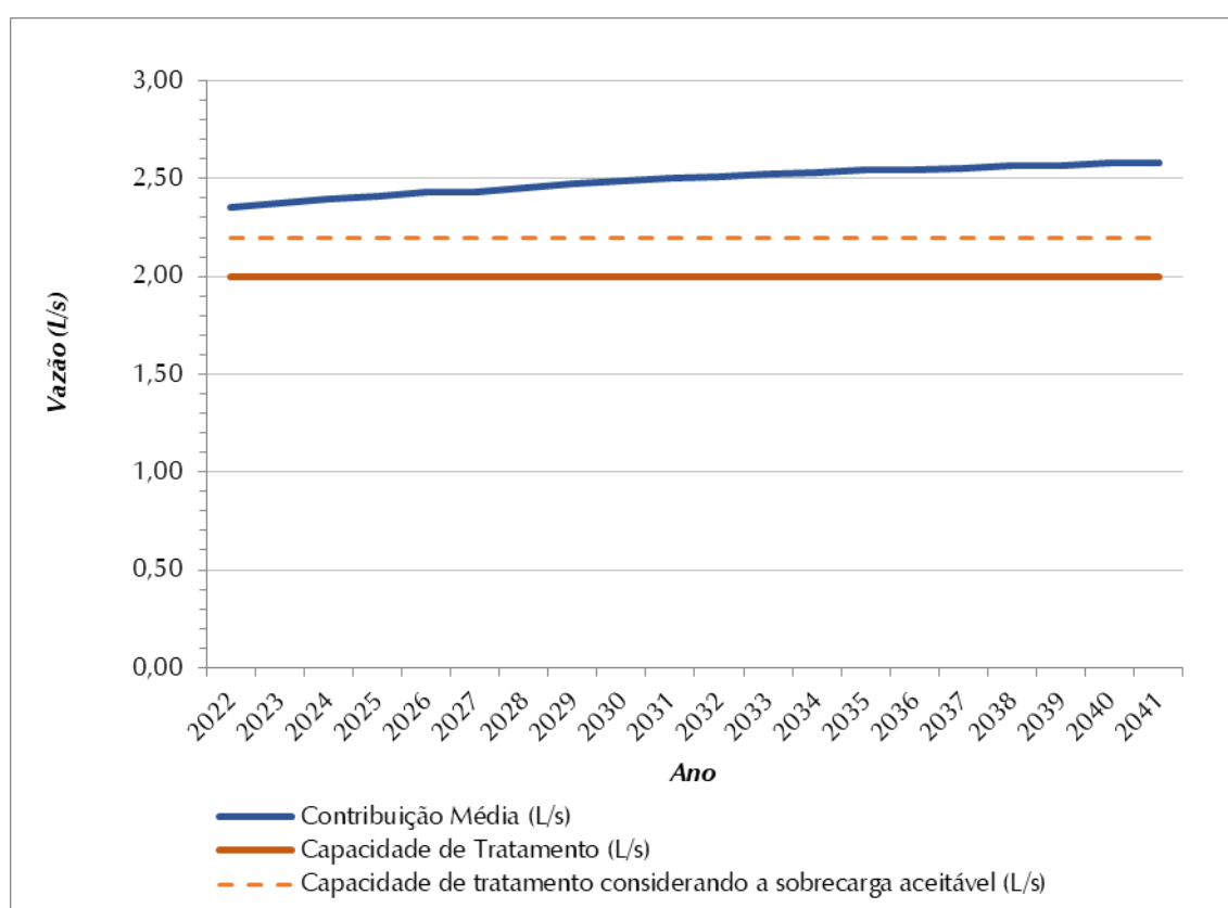
Figura 8.7 – Contribuição Média Total (L/s) x Capacidade de Tratamento de Esgoto (L/s) – SES Juritis
