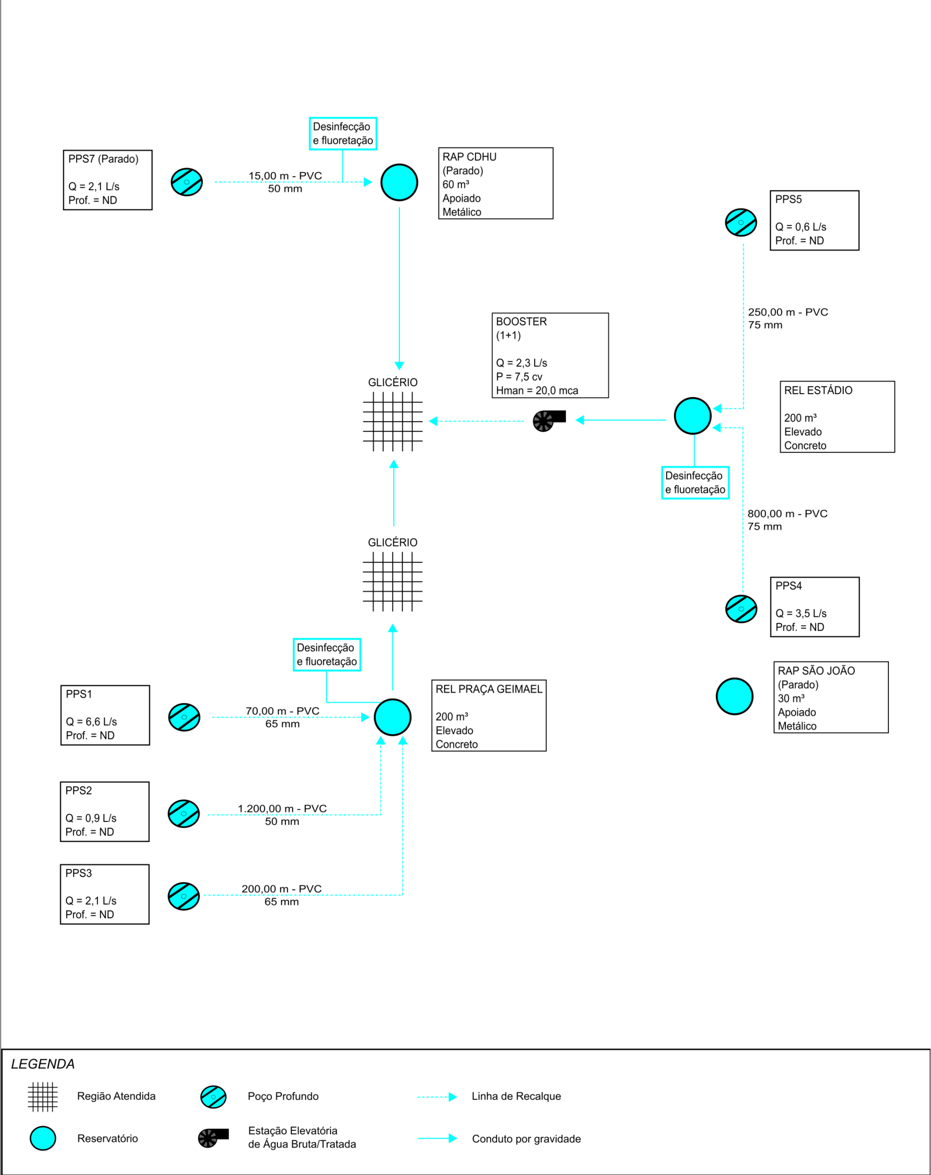
Figura 4.1 – Croqui do Sistema de Abastecimento de Água Sede
