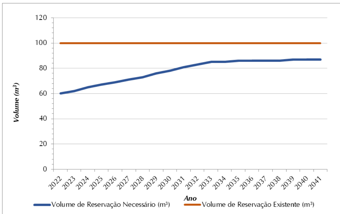
Figura 8.4 - Volume de Reservação Necessário (m³) x Volume de Reservação Atual (m³) SAA Juritis
