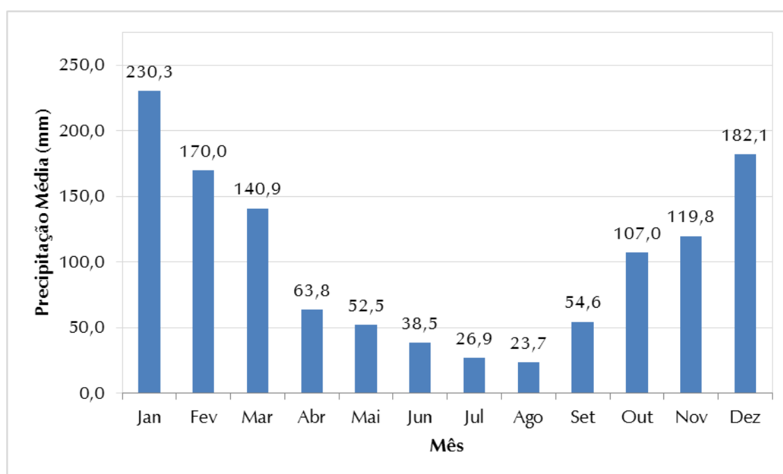
Figura 3.2 - Precipitação Média Mensal no Período de 1944 a 2021, Estação C7-024
