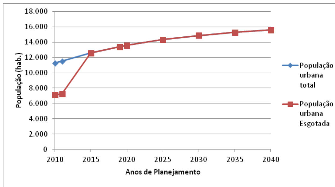
Gráfico 2.4 - População urbana total x população urbana esgotada
