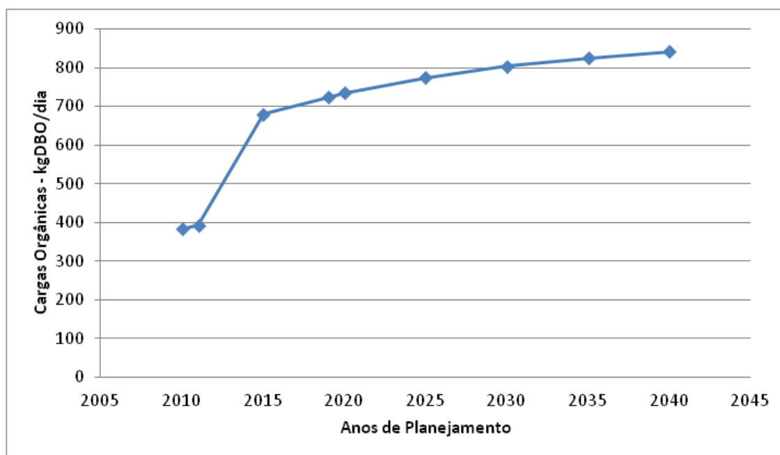
Gráfico 2.6 – Evolução das cargas orgânicas - kg DBO/dia
