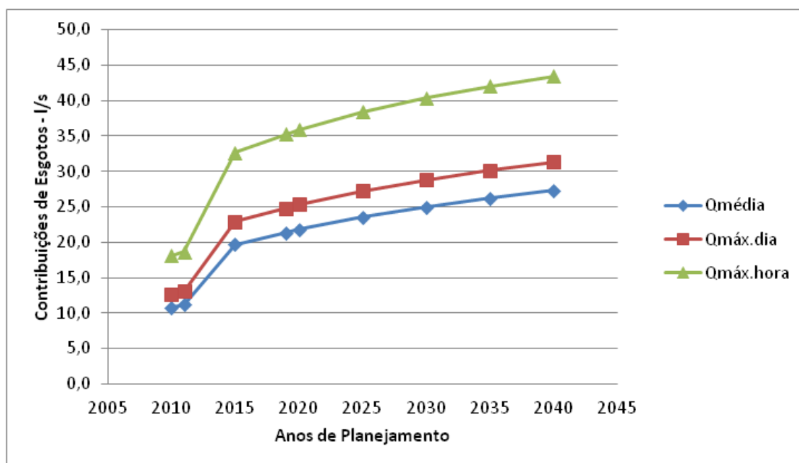
Gráfico 2.5 – evolução das contribuições de esgotos
