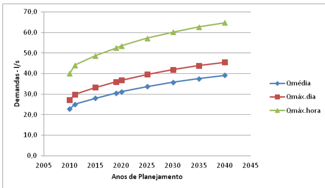
Gráfico 2.2 – Evolução das demandas/vazões disponibilizadas para distribuição
