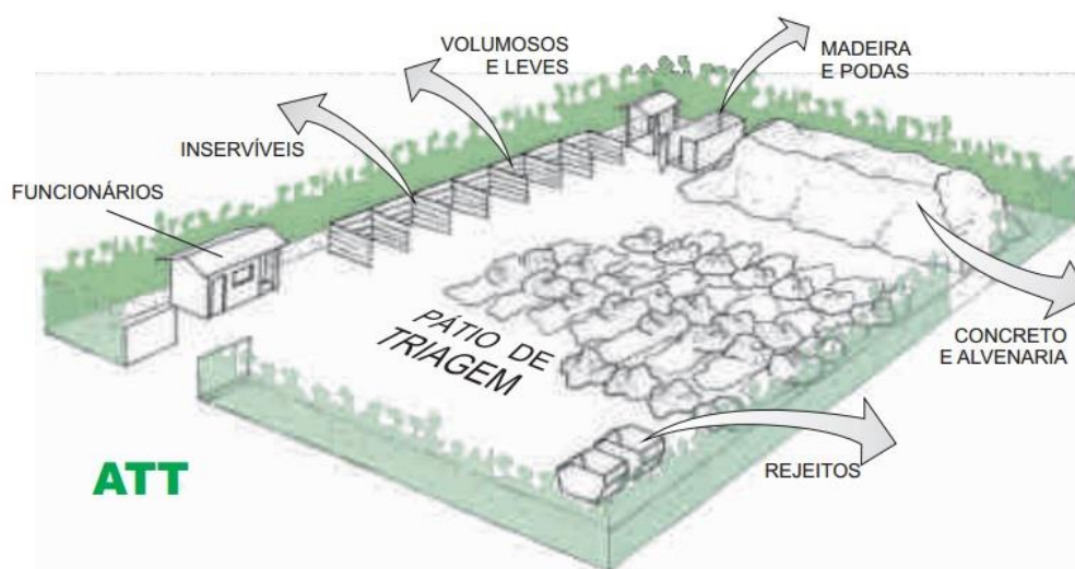
Figura 60: Modelo de Áreas de Triagem e Transbordo. Fonte: Ministério do Meio Ambiente.
