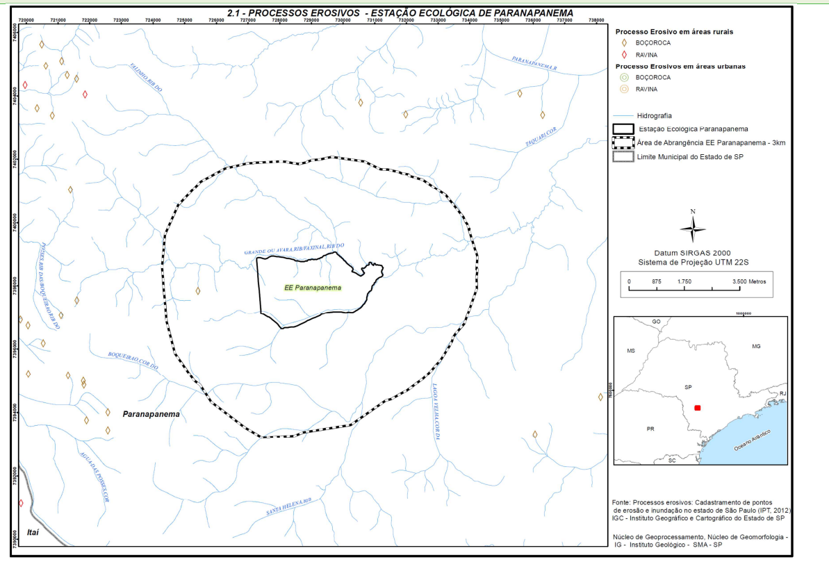
APÊNDICE 2.3.2.A Mapa de processos erosivos na Estação Ecológica de Paranapanema e entorno (dados extraído IPT, 2012)
