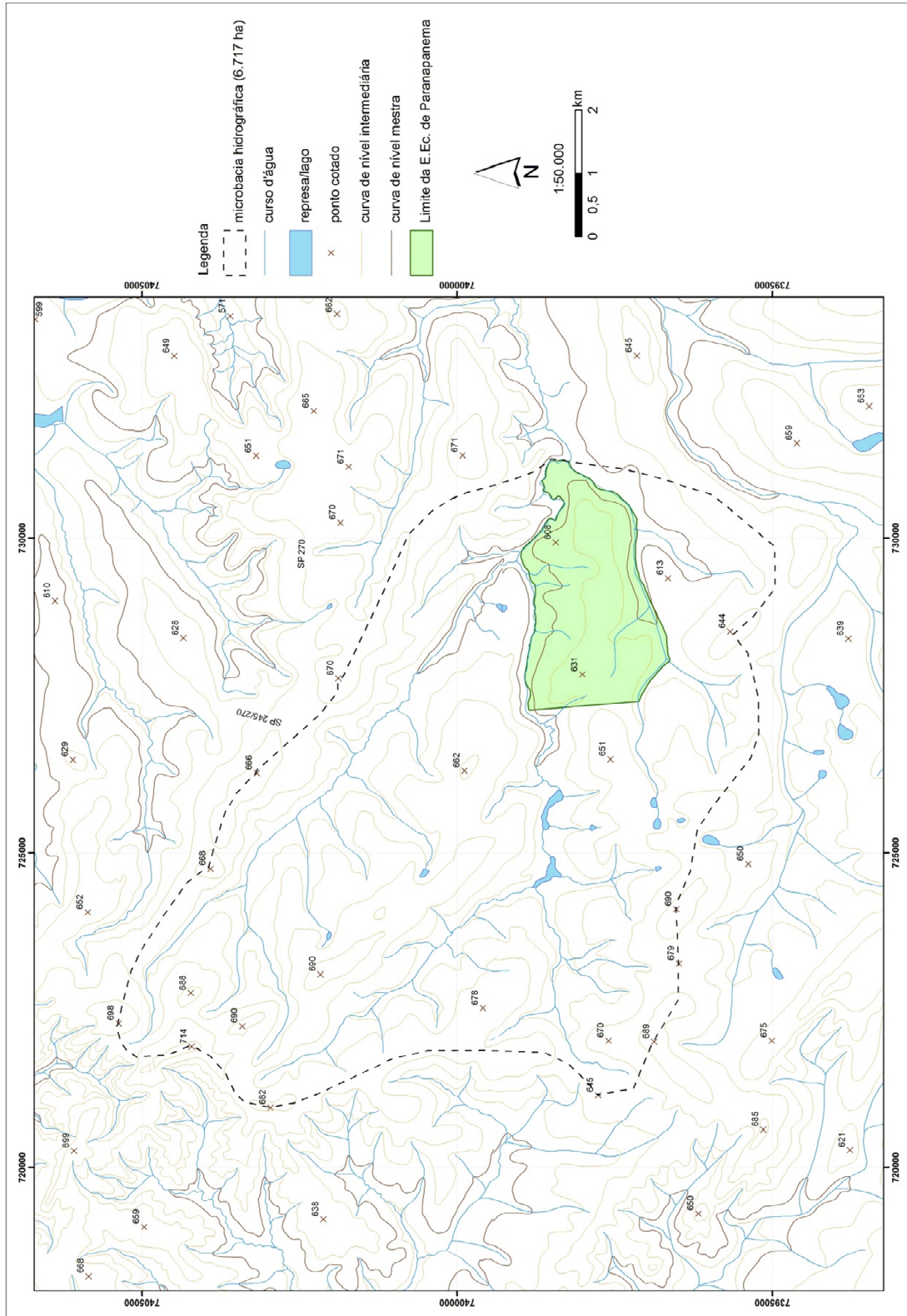
APÊNDICE 2.3.5.E. Mapa de Bacia de Drenagem na Estação Ecológica de Paranapanema e Entorno (IF, 2017)
